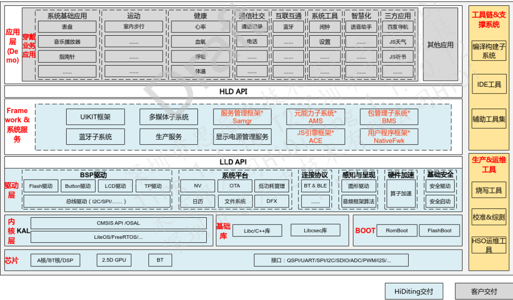
图1-1 HiDiTingV100 产品解决方案系统架构图
